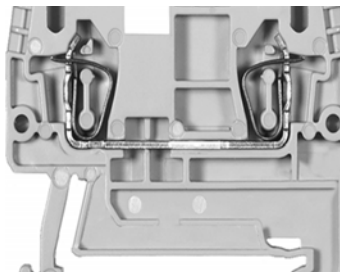
Клеммная колодка типа AB1 RRN
