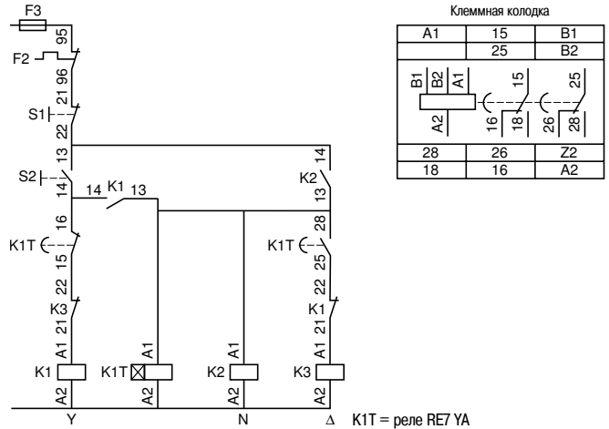
Клемная колодка
