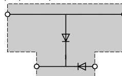
AB1 ET435U2DRO (1 А / 1000 В)
