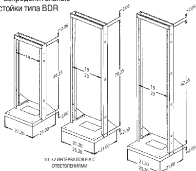
Распределительные стойки типа BDR
